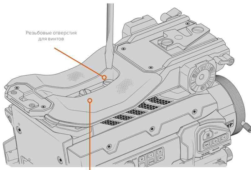
Два винта 1/4 дюйма для опорной пластины
