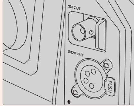
URSA Broadcast kameradaki SDI ve 12V güç bağlantıları
