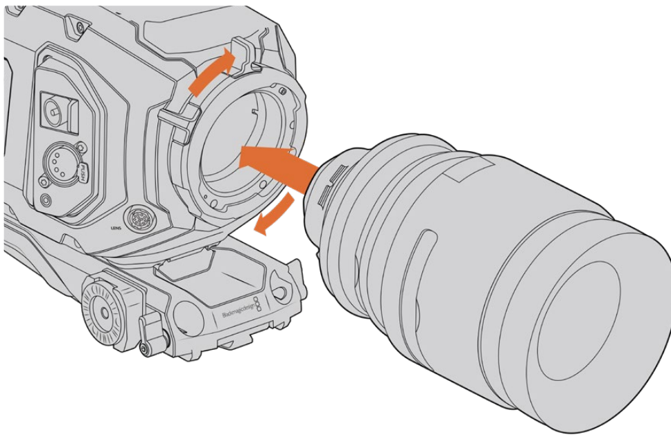
PLレンズの装着/取り外し
