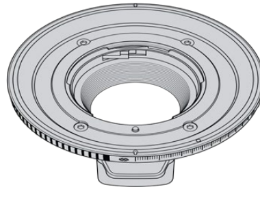
F 마운트
