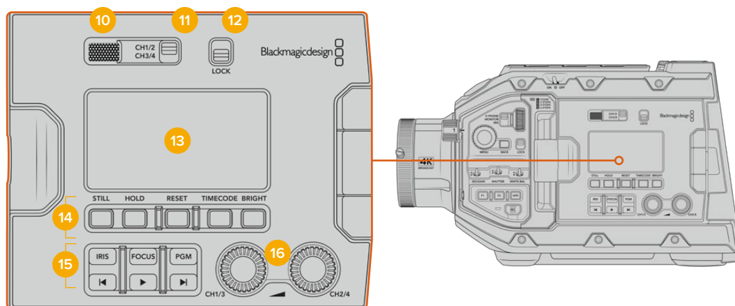
Panel de control ergonómico del modelo URSA Broadcast
