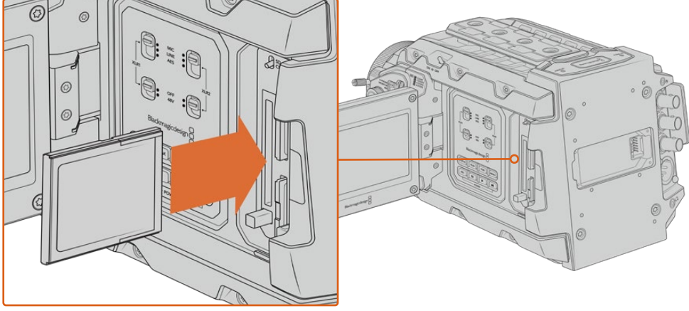
Blackmagic URSA Broadcast, aralıksız kayıt için iki CFast yuvaya sahiptir.
