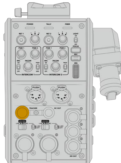
Takipçi Arayüzü (Tracker Interface) konektörü
