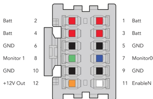
Vista posteriore degli alloggiamenti dell'adattatore. Consulta la tabella di configurazione dei fili per la descrizione di ogni alloggiamento
