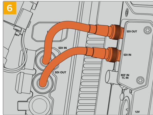
6 同梱のBNCケーブルでカメラの背面のSDI出力をBlackmagic Camera Fiber ConverterのSDI入力に接続し、Camera Fiber ConverterのSDI出力をカメラの背面のSDI入力に接続します。
