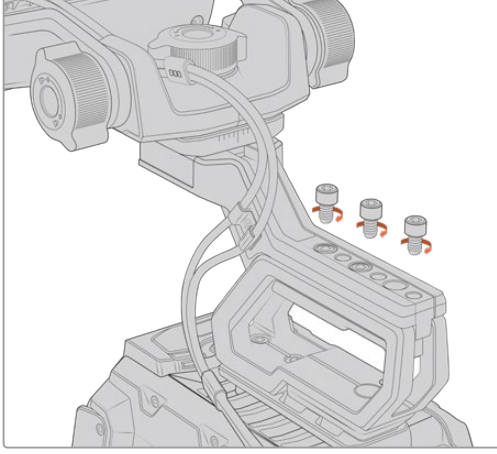
Blackmagic URSA Studio Viewfinder, omuzda çekim aparatına bağlıyken
