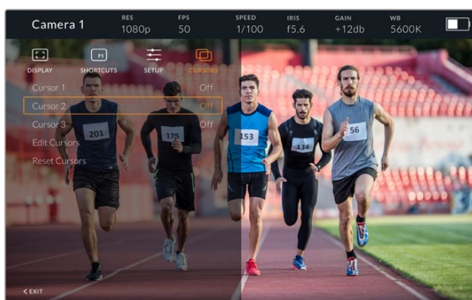
Меню Cursors
