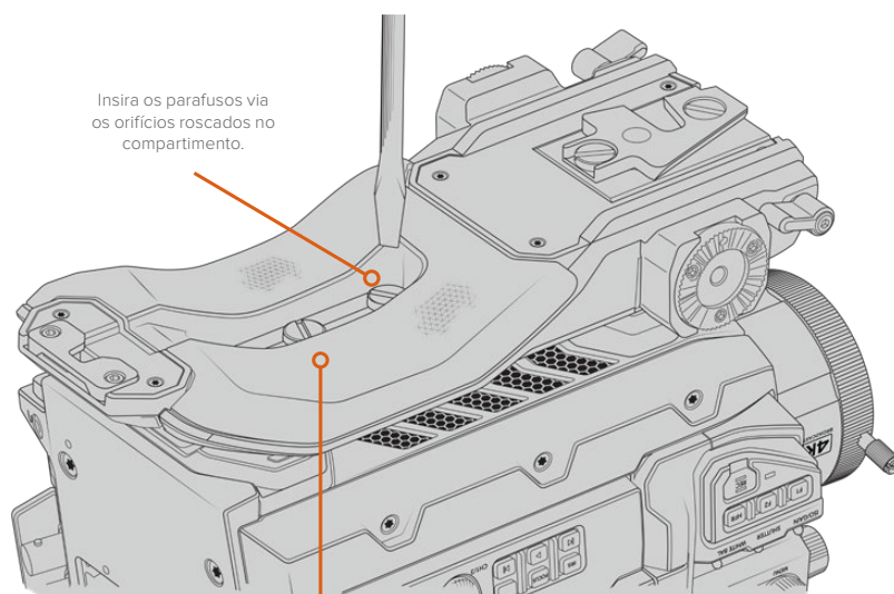
2 x parafusos de 1/4" para a placa de base
